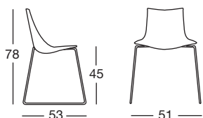
Struttura a slitta Sledge frame Art. 2265
