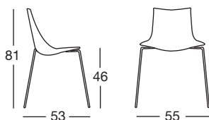
Struttura a 4 gambe 4-leg frame Art. 2266
